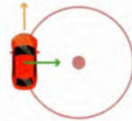
32 centripetal force 向心力
