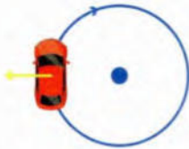
31 centrifugal force 离心力
