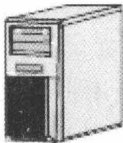
Web服务器
