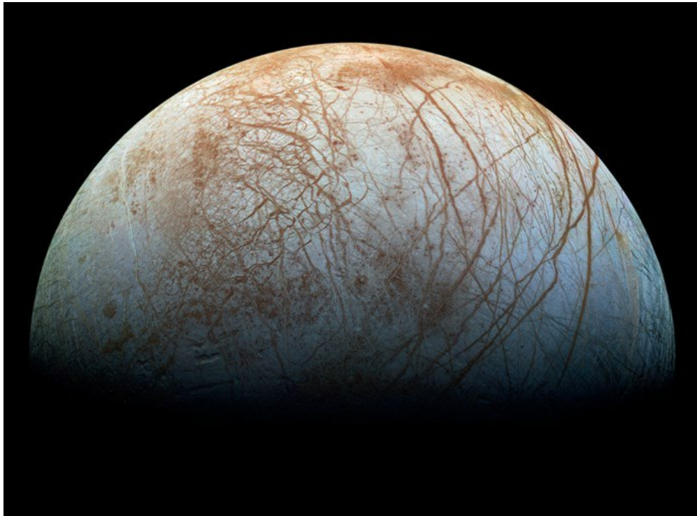
1997 年伽利略号探测器观测到的木卫二，冰壳显示出惊人的纹路，
