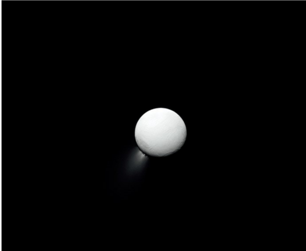
2012 年卡西尼号探测器拍摄的土卫二，可见往外喷出的水
